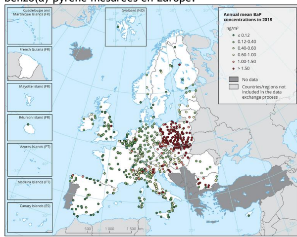
Figure 1 : concentrations de benzo(a)-pyrène mesurées en 2018 en Europe (AEE 2020)
