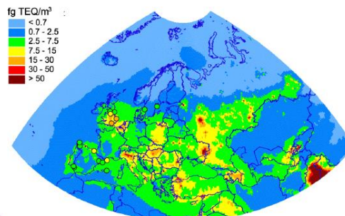
Figure 2 : Distribution spatiale des concentrations de dioxines et furannes modélisées à partir de données de concentrations et d'inventaires d'émissions ajustés dans la zone EMEP en 2016 (EMEP 2018) en 2016 dans la zone EMEP (AEE 2018)
