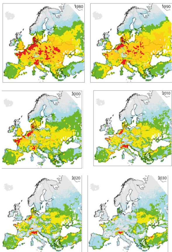
Figure 1 : Dépassement moyen cumulé des charges critiques calculées pour l'eutrophisation de 1980 à 2020 en vertu du Protocole de Göteborg amendé de 2012 (scénario GP-CLE) et en 2030 sous un scénario de réduction maximale réalisable (MAAS 2016).
