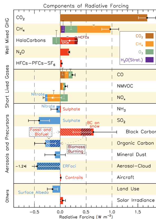
Figure 5 : Forçage radiatif des composés (IPCC- AR5-2014).
